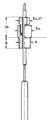
9 - Branchement mâle tournant et coulissant
